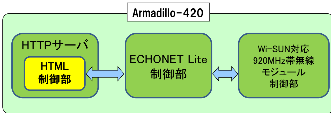
図1 コントローラ概略ブロック図
